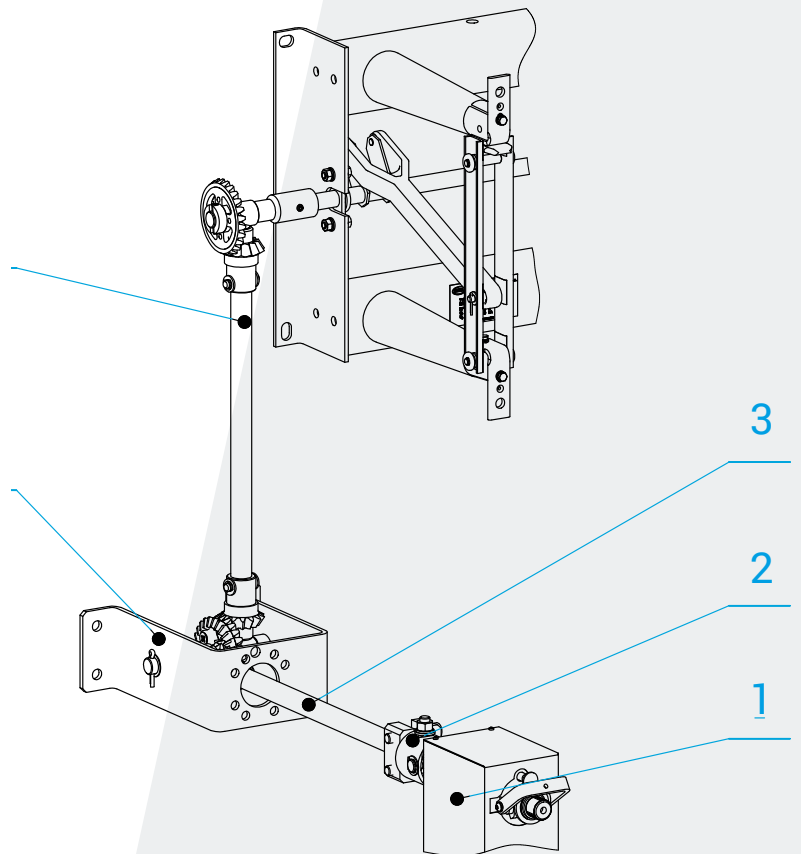
Zeichn. 11. Verbindung des Trennschalters mit dem Winkelgetriebe.
