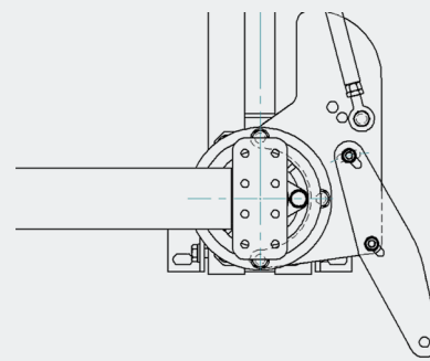
Dźwignia regulacyjna – położenie neutralne
